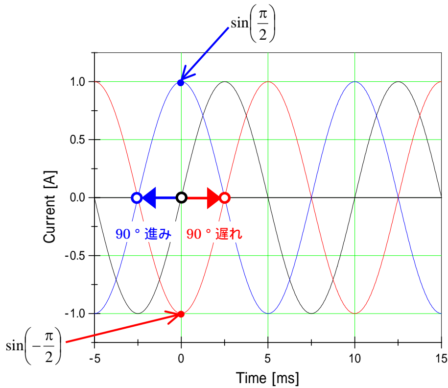
図1 3種類の位相差の正弦波波形 (—: 0 rad、—: 位相角 -\pi/2 rad、—: 位相角 \pi/2 rad)
