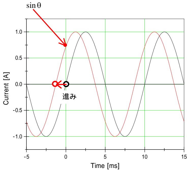
図2 2種類の位相差の正弦波波形 (—: 0 rad、—: 位相角 \theta rad)
